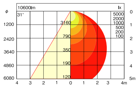
1/2照度角図及び直射水平照度分布図
