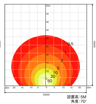
1/2照度角図及び直射水平照度分布図
