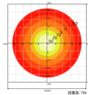
1/2照度角図及び直射水平照度分布図
