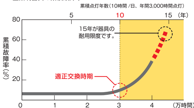
■照明器具の累積故障率
